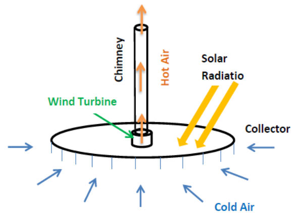
Fig. 8- Solar Chimney
